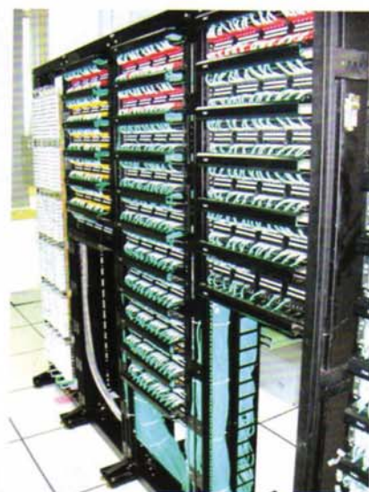
綜合佈線完工機架圖
